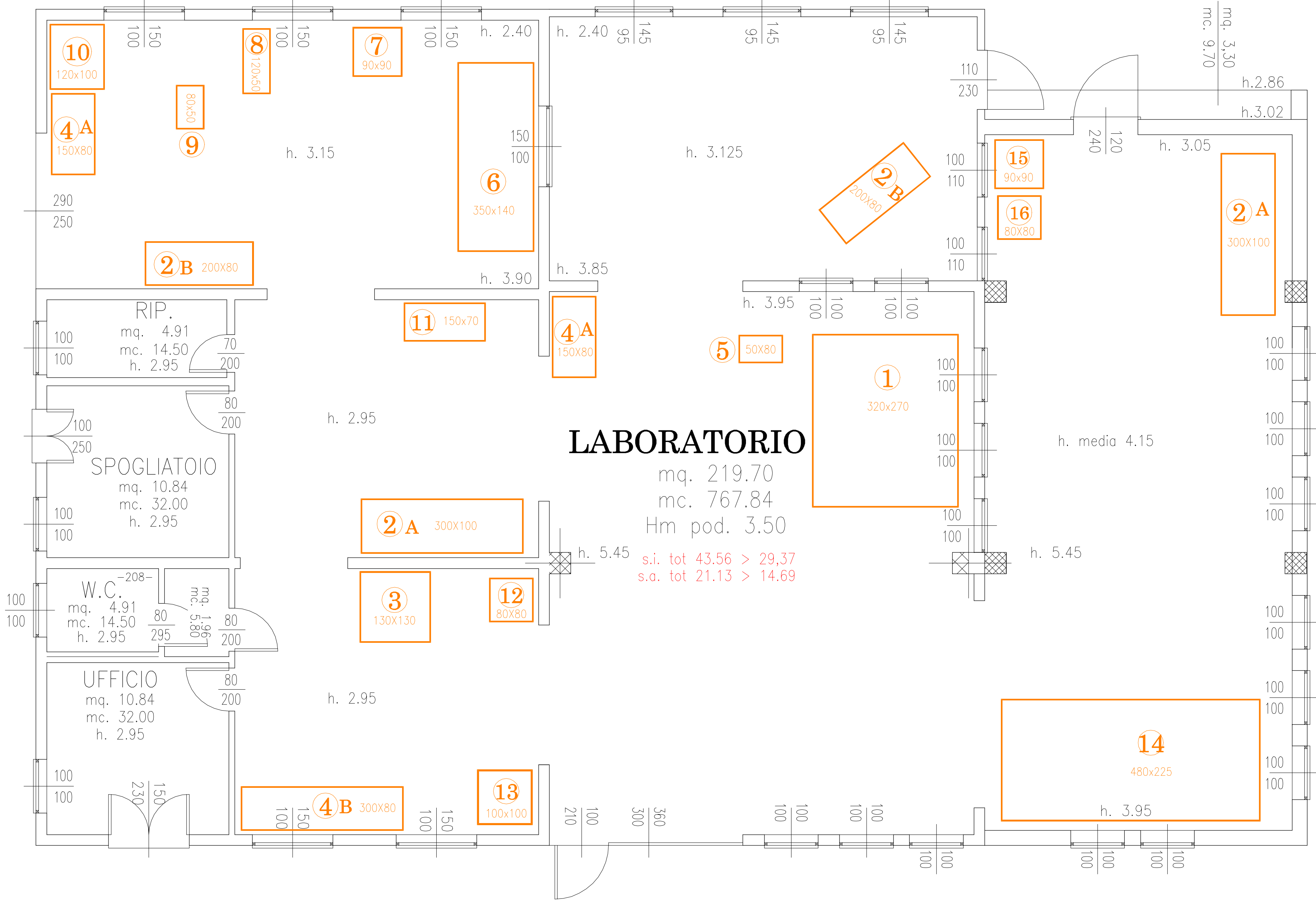
PIANTA LAYOUT ACCESSORI SCALA 1:50
